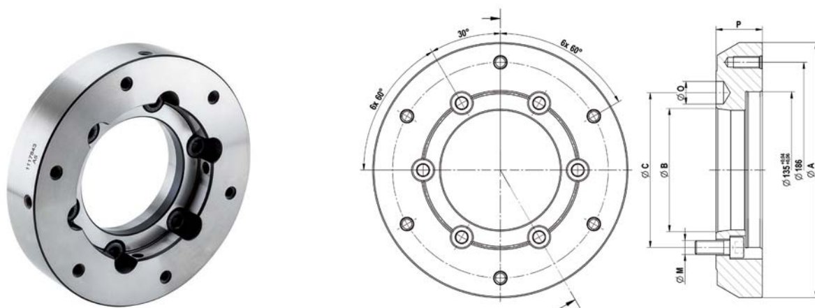
C 18 Zwischenflansch ISO 702-1 (DIN 55028)
