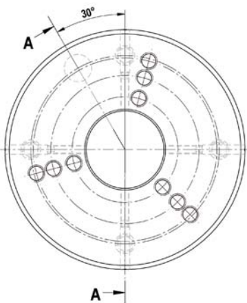
C 18 Zwischenflansch ISO 702-3 (DIN 55027/55022) mit Einstellschrauben
