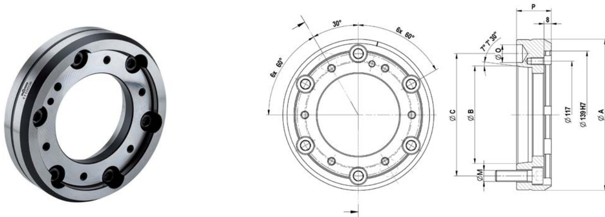
C 18 Zwischenflansch ISO 702-1 (DIN 55028), für Größe 00-04
