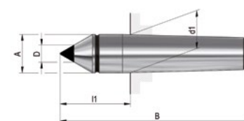
A07 DIN 806, full point, material: tool steel
