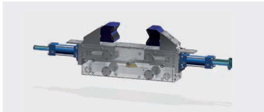
Zentrischspanner, Hub pro Backe 175 mm
