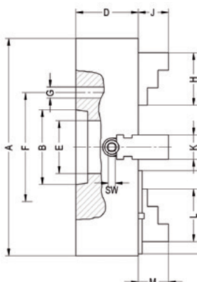
DIN 55026 mounting from front 1) Not for DIN 55021 or A1/A2 inch 2) Not for A1/A2 inch
