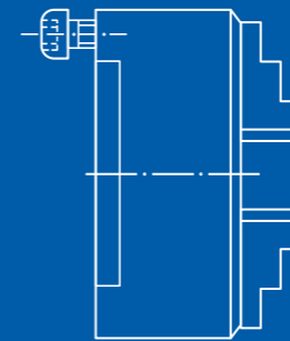
DIN6350, forma A para la atornilladura posterior
