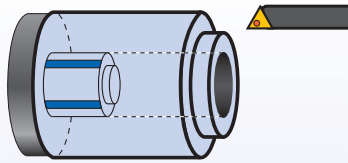
WERKSTÜCK Flansche
